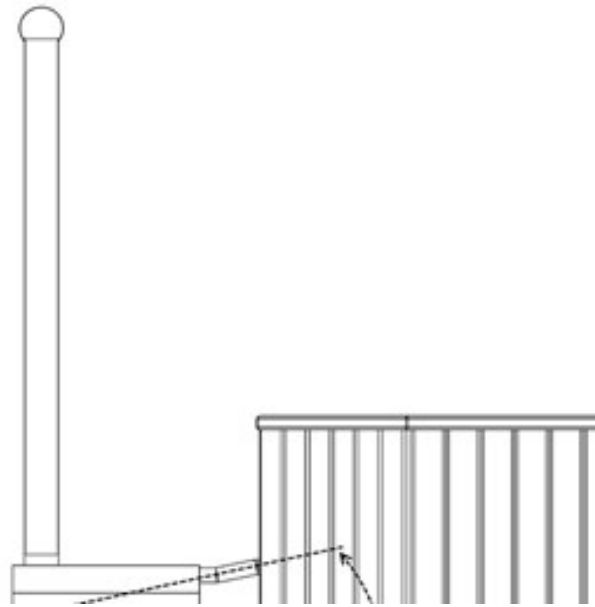
Bild 3. Korrekt placering av elastiska slangar vid anslutning av kaminen till badtunnan
