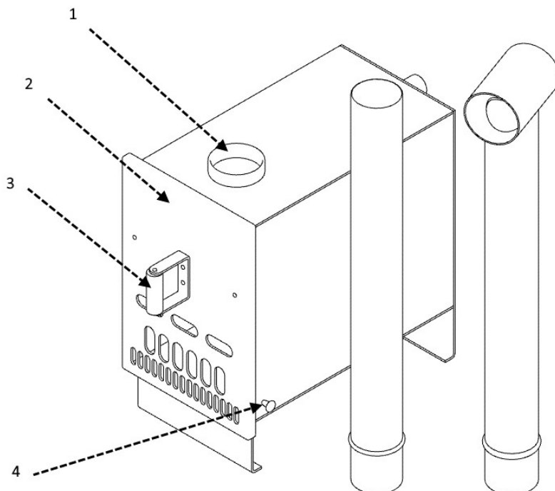
Bild 2. Komponenter av den externa kaminen
