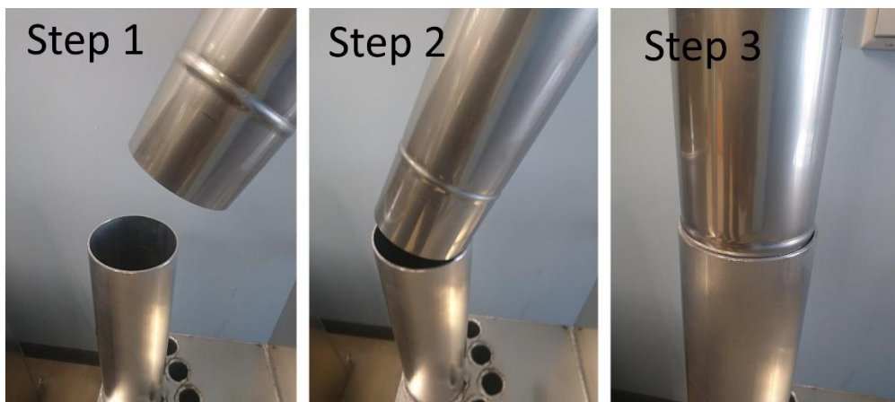
Bild 3. Montering av skorstenen
